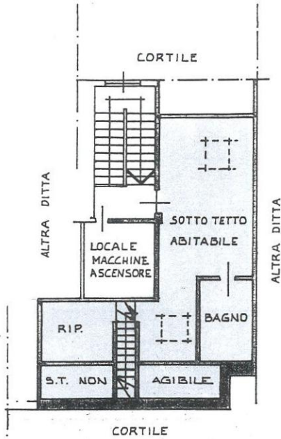
PIANTA PIANO SOTTOTETTO (Hm = 2,10 mt.)
